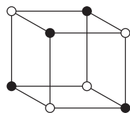
食盐晶体的微观结构
